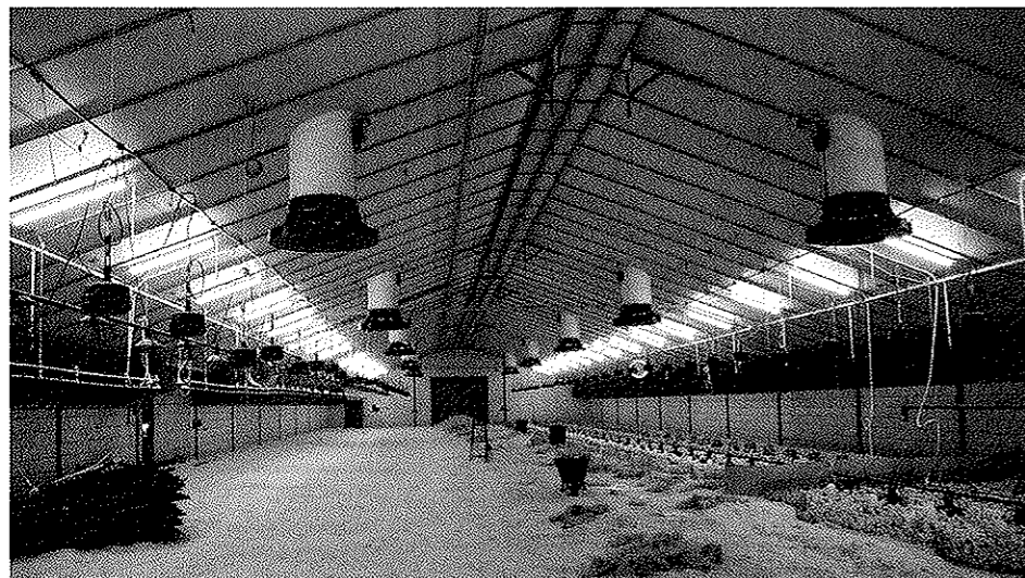
In het dak van de opfokstal zijn, in twee rijen, 18 kunststof kokers geplaatst. Per koker is 10.500 m 3 ventilatiecapaciteit geïnstalleerd. In de kokers zit een speciale ventilator, een klep en een venturiring
